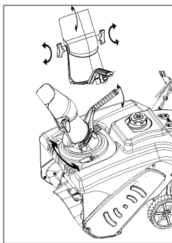
Рис. 10 Управление желобом снегоотбрасывателя
